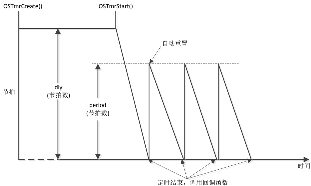
图 9.1.4 周期定时器( dly>0, period>0 )
