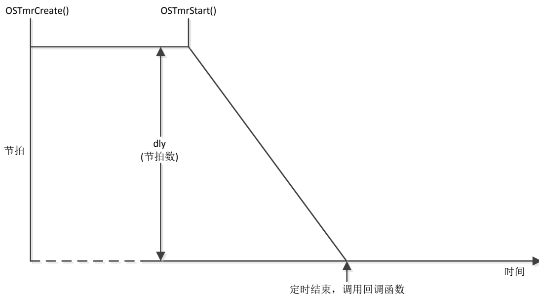
图 9.1.1 单次定时器
