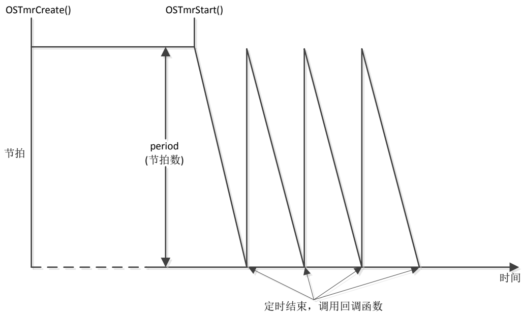
图 9.1.3 周期定时器 ( dly=0, period>0 )
